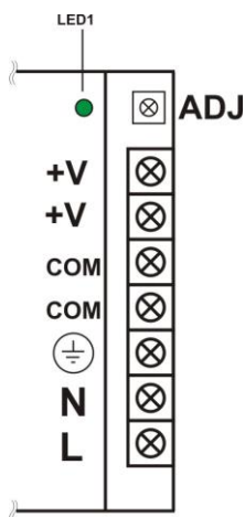
Abbildung 1. Beschreibung der Netzteilstöße.
