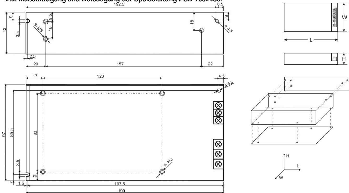
Abbildung 2. Mechanische Ansicht der Speiseleitung.
