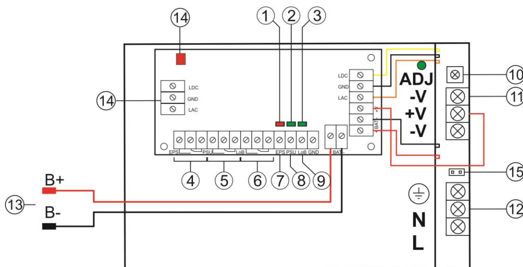
Abbildung 3. Ansicht der Speiseleitung mit dem Modul MPSB24.
