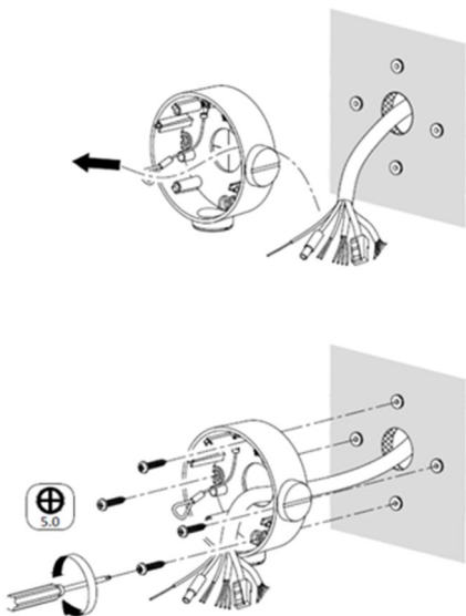
Abbildung 2-3 Kabel anschließen
