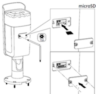
Abbildung 2-1 Speicherkarte einsetzen
