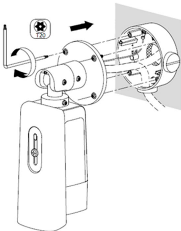
Abbildung 2-5 Kamera befestigen
