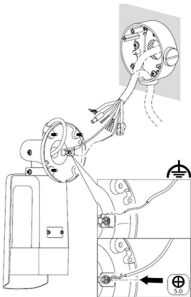
Abbildung 2-4 Sicherheitsseil befestigen
