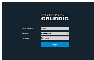
Abbildung 3-1 Login Oberfläche
